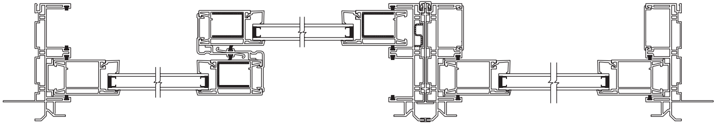
Slide Patio Door 3 Wide - Horizontal Section
