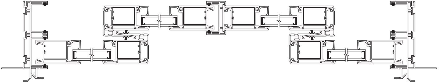
Slide Patio Door OXXO - Horizontal Section
