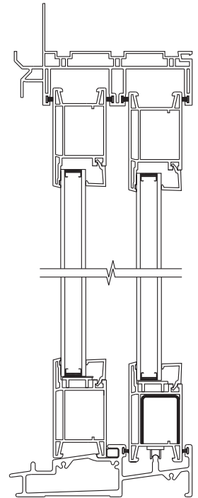
Slide Patio Door Vertical Section
