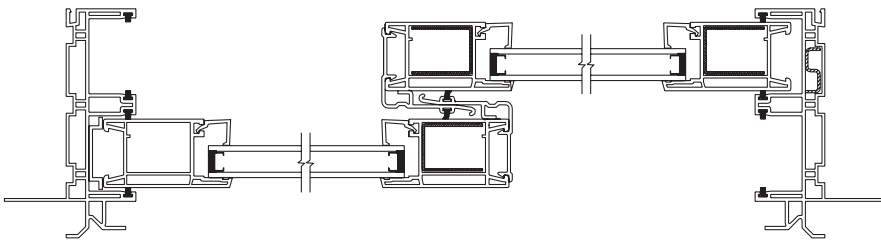
Slide Patio Door Horizontal Section
