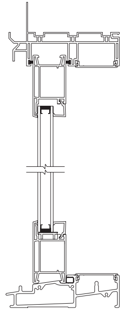
Slide Patio Door Sidelite - Vertical Section
