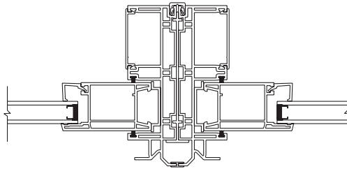
Slide Patio Door Sidelite - Horizontal Section
