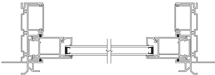
Slide Patio Door Sidelite - Horizontal Section
